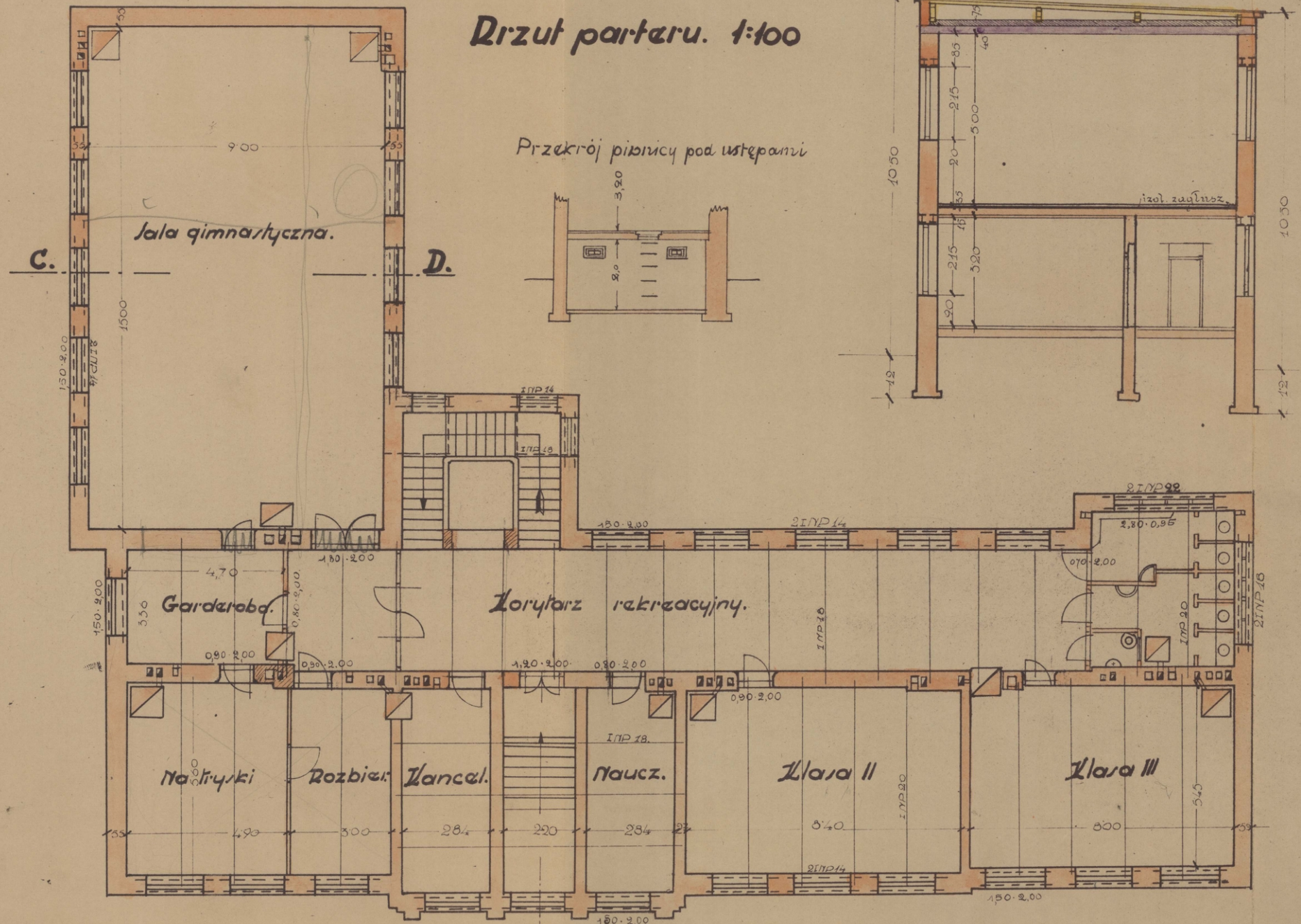
Fragment planu architektoniczno-budowlanego Domu Pereca, wyk. inż. H. Bekker, 1938 (APL, Akta Miasta Lublina, Inspekcja Budowlana, sygn. 721)
